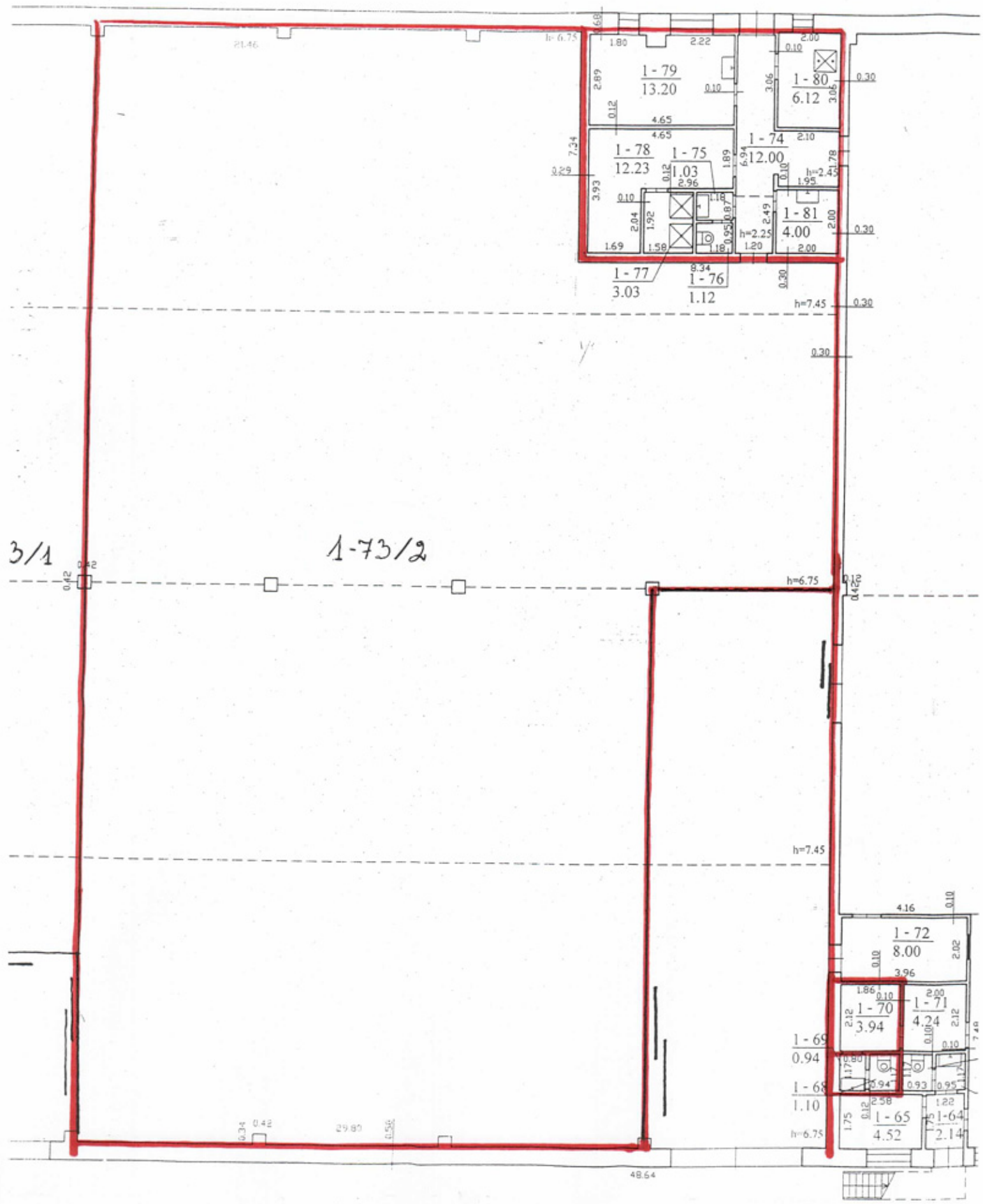
PIRMO AUKŠTO PLĀNAS
